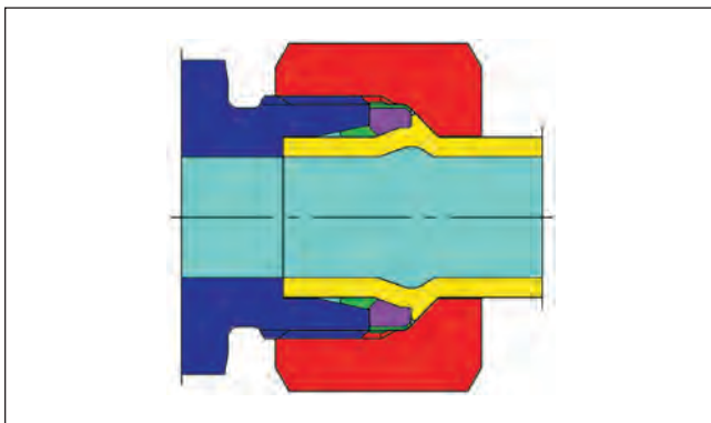
La nueva conexión EO2-FORM: Extrema rigidez y bajos pares de apriete
